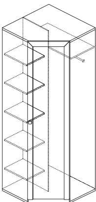
■ СП.0111.405 Шкаф угловой (дверь глухая в комплекте) (ВхШхГ): 2267 x (909 x 909) x 590
