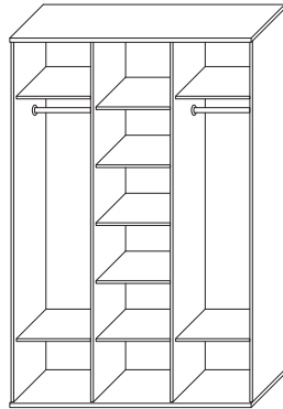
■ СП.013.403 Шкаф 3-х дверный (корпус) (ВхШхГ): 2217 x 1450 x 574
