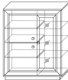
2 ГТ.0114.302 Шкаф 3-х дверный (1 стеклодверь) 1179 низкий (ВхШхГ): 1425 x 1179 x 426
