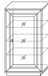
14 ГТ.0114.306 Шкаф (1 стеклодверь) 776 низкий (ВхШхГ): 1425 x 776 x 426
